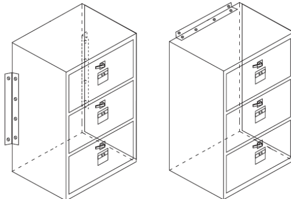
Figure 53 : Exemples de meubles classeurs renversés, et de sécurisation. (Source FEMA)
