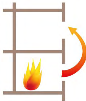
Figure 57 : Schéma indiquant la possibilité inacceptable de transmission d'un incendie d'un étage à l'autre par la façade. (Source ANCO/PAHO)
