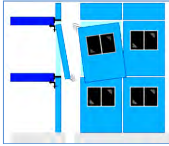
Figure 34 : Illustration schématique de la rupture de fixations d'un panneau de façade préfabriqué par manque d'adaptation aux déformations de la structure pendant un séisme. (Source ANCO)
