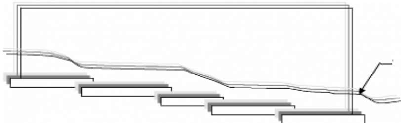
Figure 16 : Semelles décalées sur site en pente (principe schématique). (Source ANCO)
