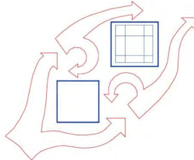
Figure 59 : Effet de masque par des bâtiments en amont du sens du vent : La localisation de certains bâtiments peut réduire l'effet des vents cycloniques sur les bâtiments environnants.
