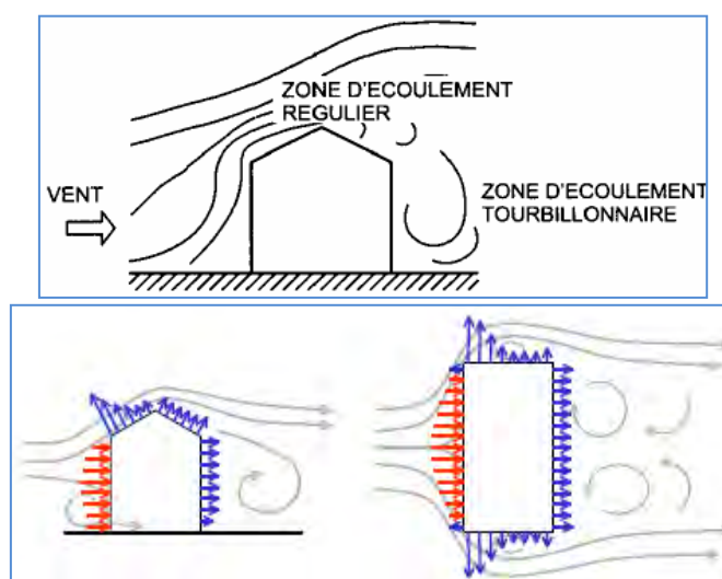
Figure 49 : Représentation schématique de l'écoulement du vent à la rencontre d'un obstacle, comme un bâtiment. (Source ENSAM)
