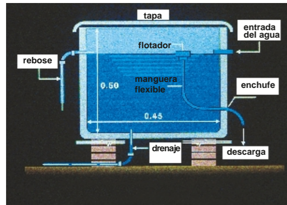
Hipoclorador simple
