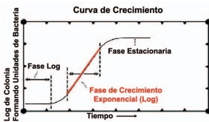
Figura 4.3—Plot de un crecimiento de fase log
